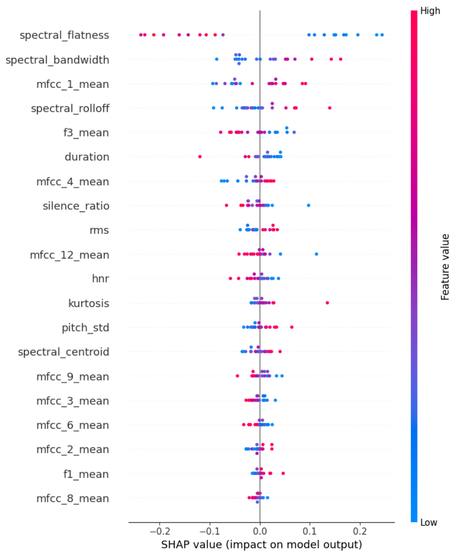
Figura 54: Explicación global con SHAP
